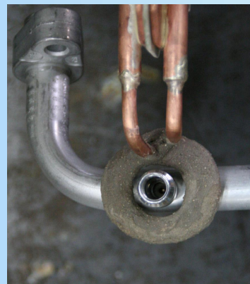
↑アルミパイプ分岐管 ロー付 平面写真
